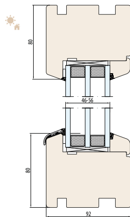
NATURO 92-FIX SYSTEEM geen afsnijding onder het raamkozijn
