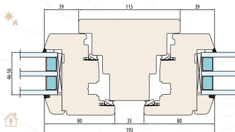
NATURO 92 SYSTEEM vaste stijl 115 mm (horizontaal doorsnede)
