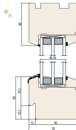
NATURO 92-FIX SYSTEEM externe afsnijding onder het raamkozijn
