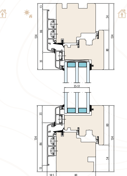
NATURO 80 ALU SYSTEEM GEMINI CLASSIC interne afsnijding onder het raamkozijn
