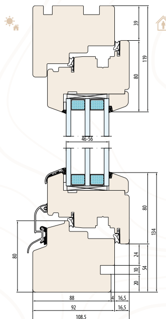
NATURO 92 SYSTEEM interne afsnijding onder het raamkozijn
